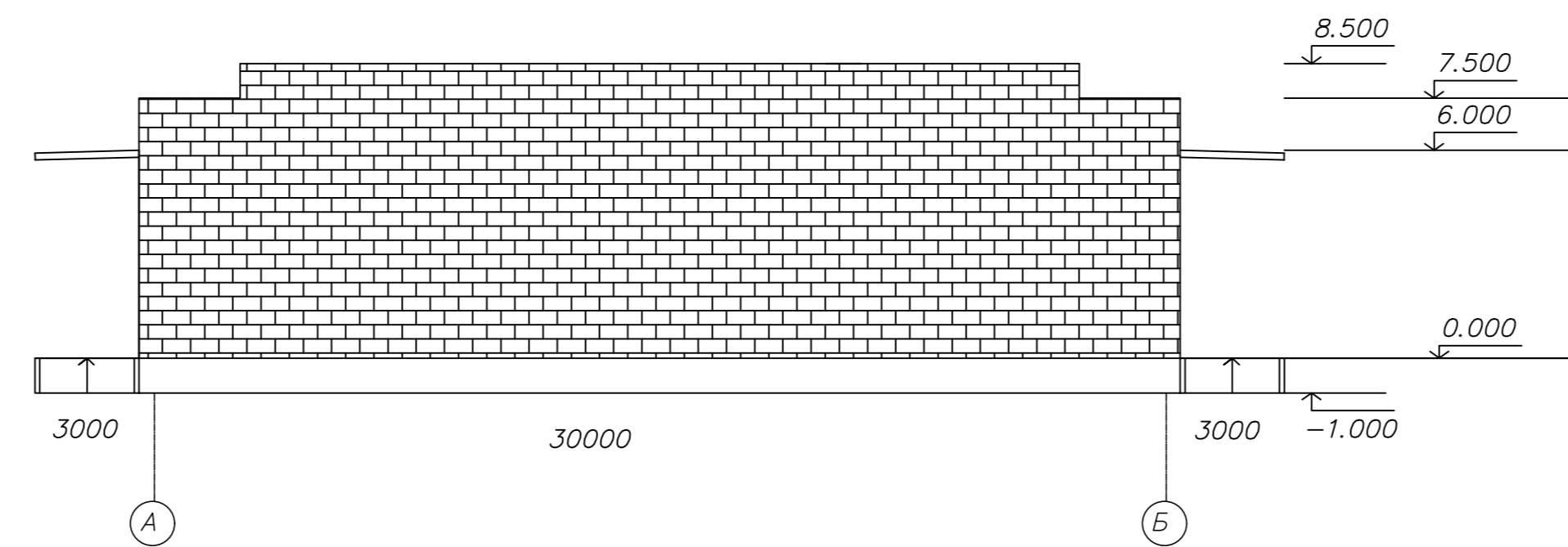
Фасад по оси А-Б
