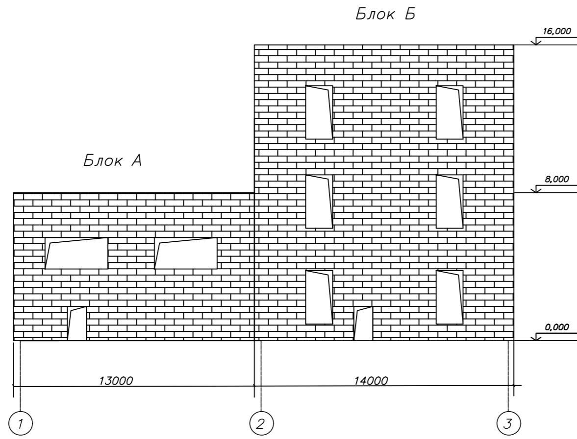
Фасад по оси 1-3
