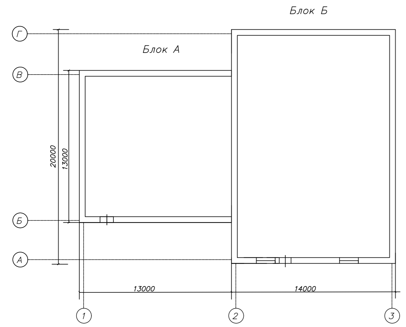
План на отметке 0.000
