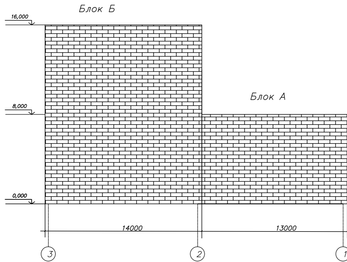
Фасад по оси 3-1
