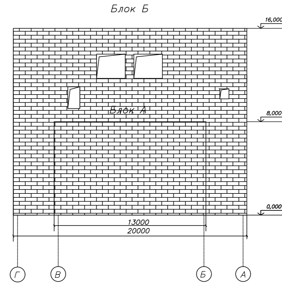
Фасад по оси А-Г
