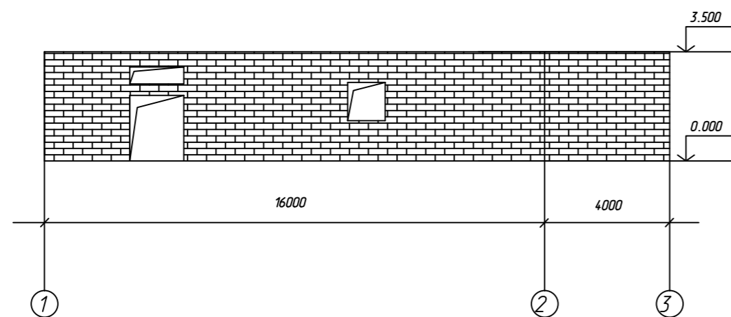
Фасад по оси 1-3
