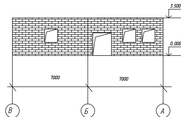
Фасад по оси B-A
