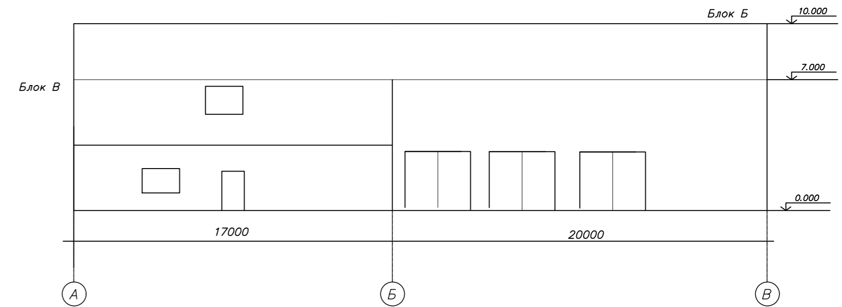
Фасад по оси А-В
