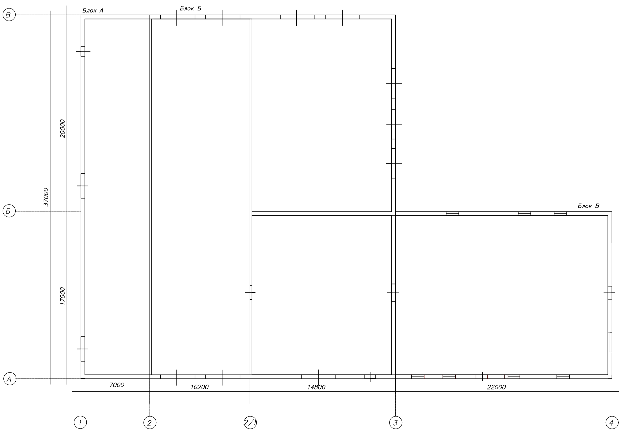
План на отм. 0.000
