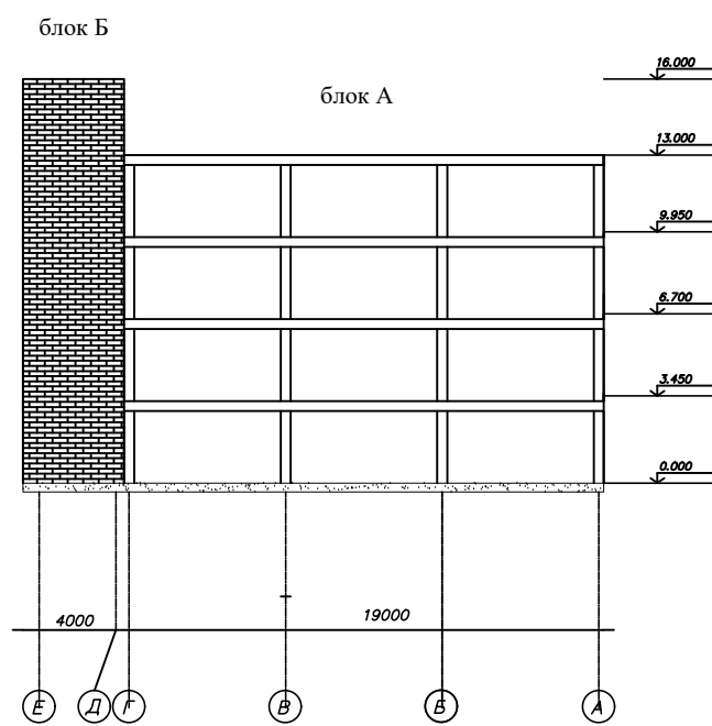
Фасад по оси Е-А
