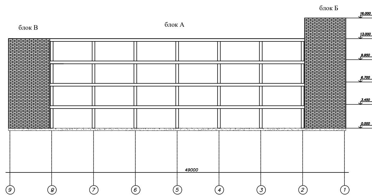
Фасад по оси 9-1
