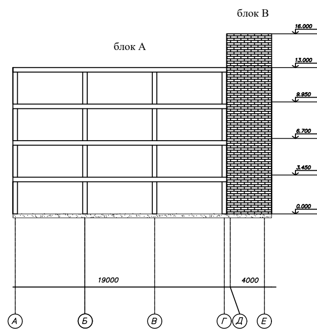
Фасад по оси А-Е
