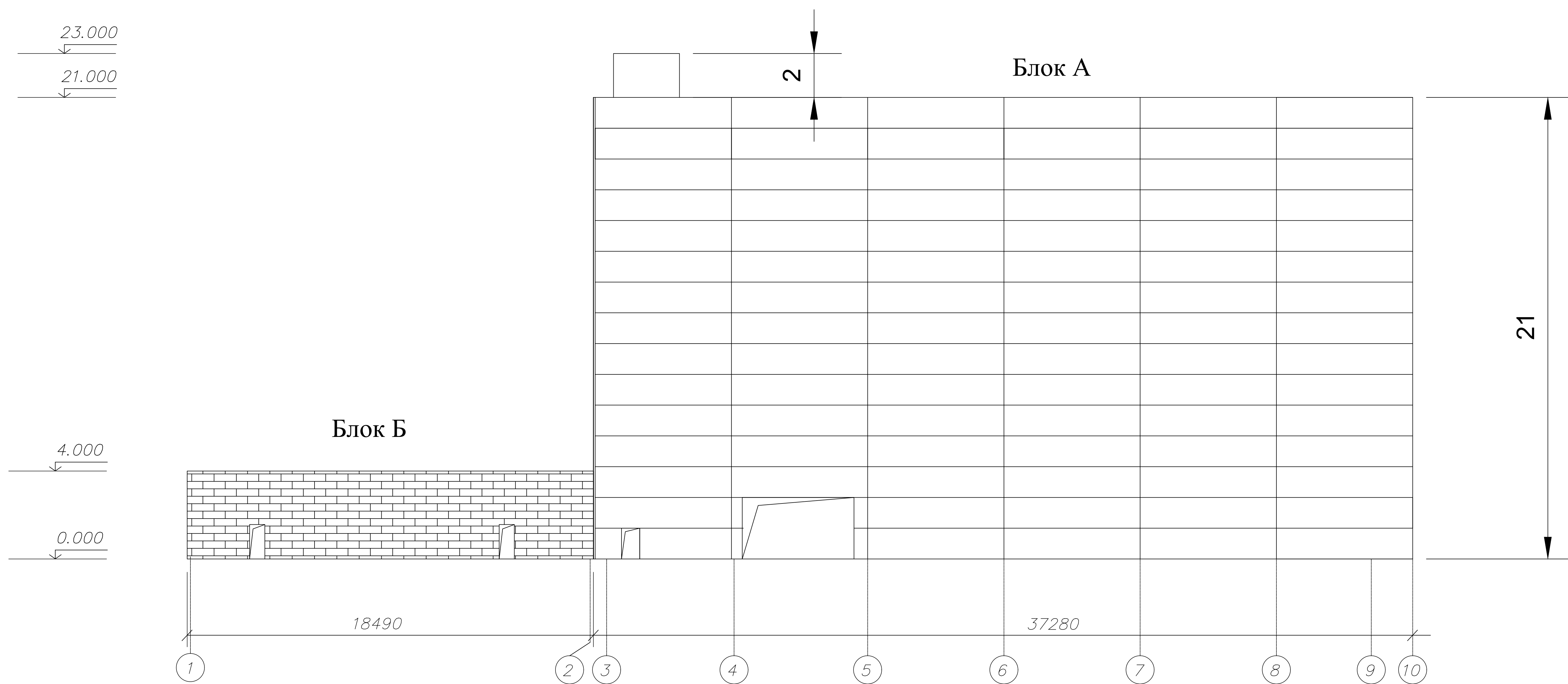
Фасад по оси 1-10
