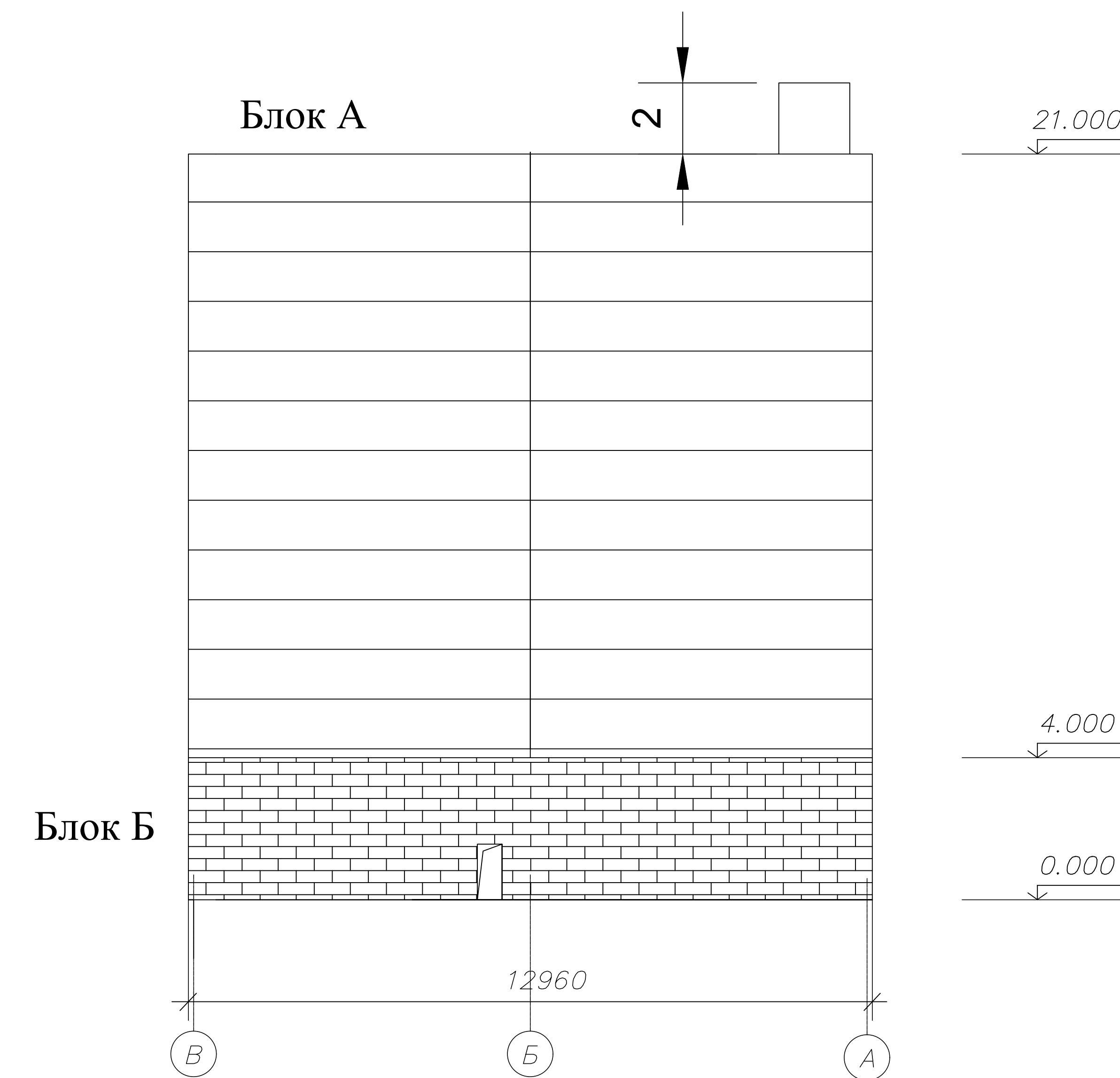
Фасад по оси В-А
