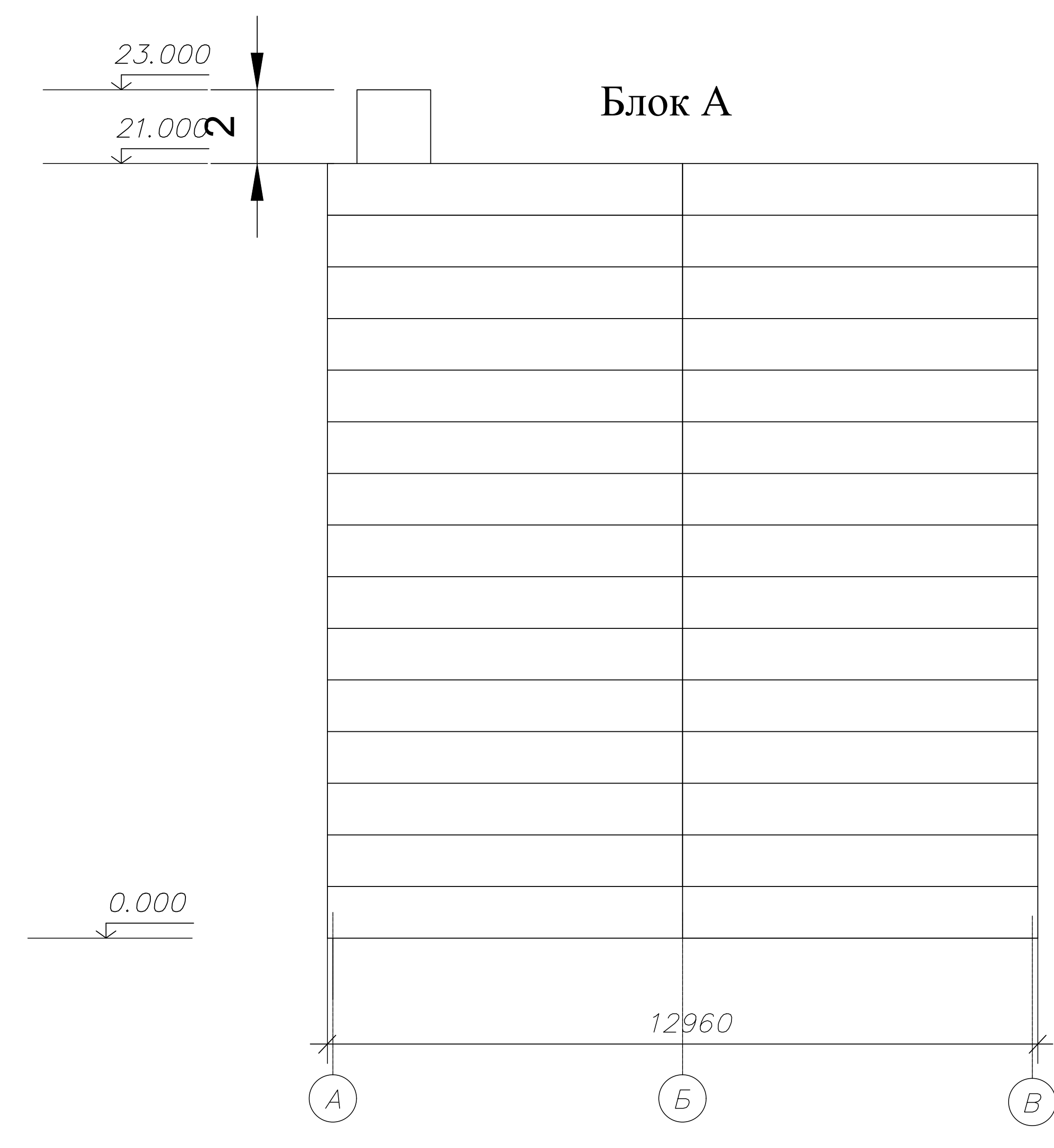
Фасад по оси А-В
