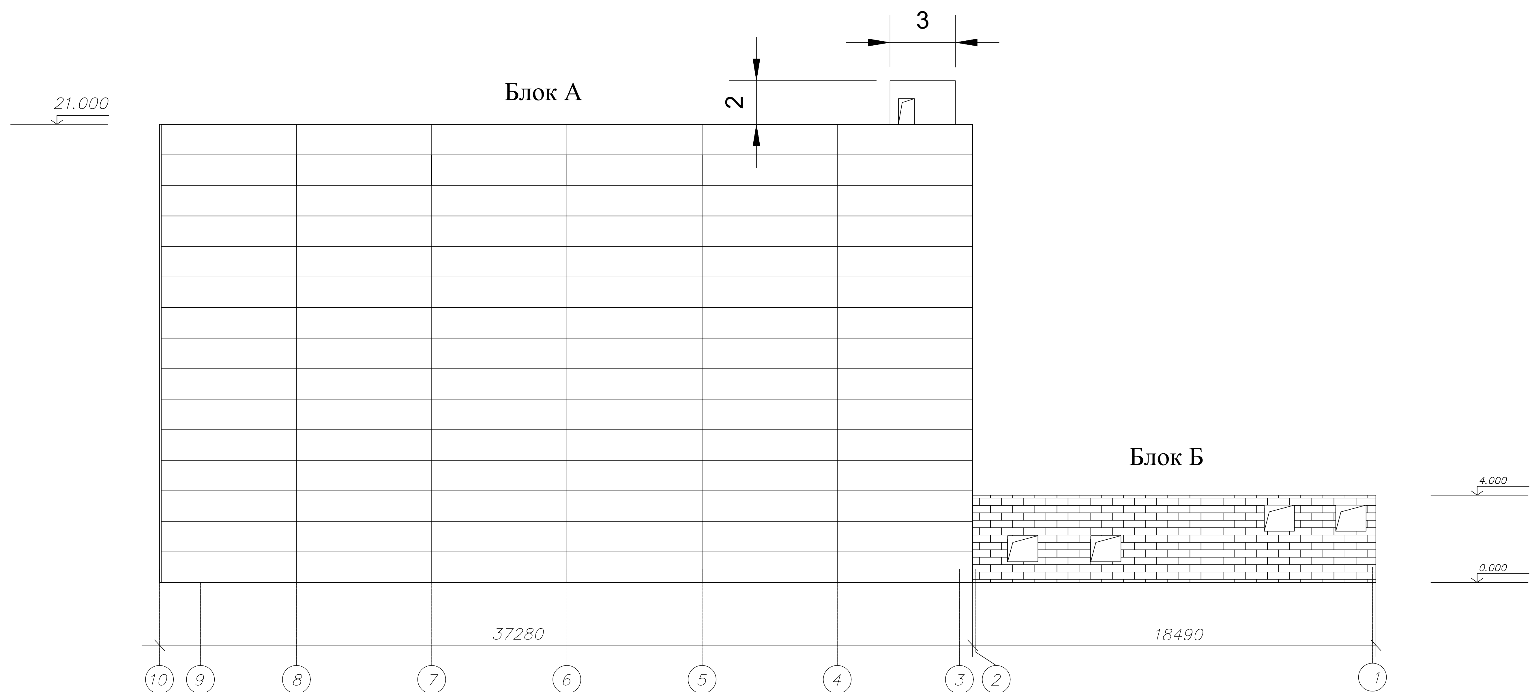
Фасад по оси 10-1
