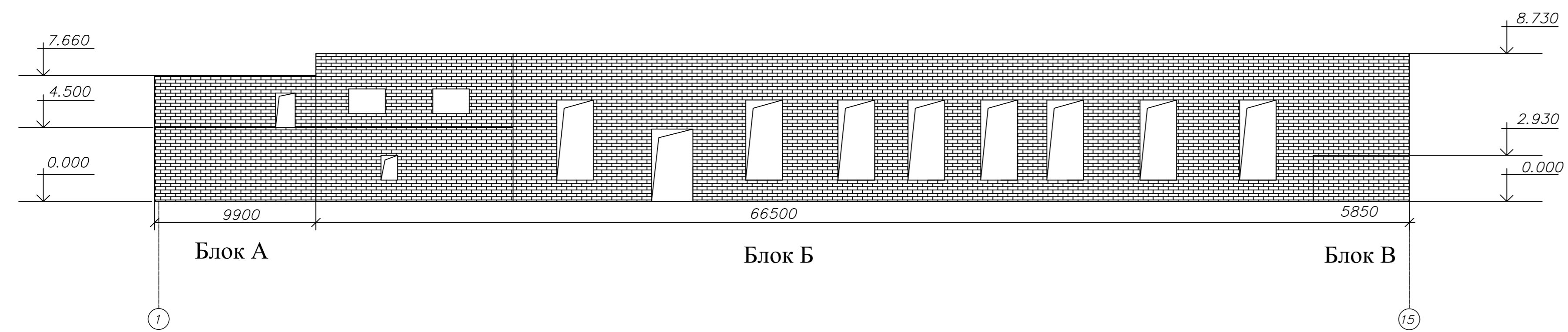
Фасад по оси 1-15
