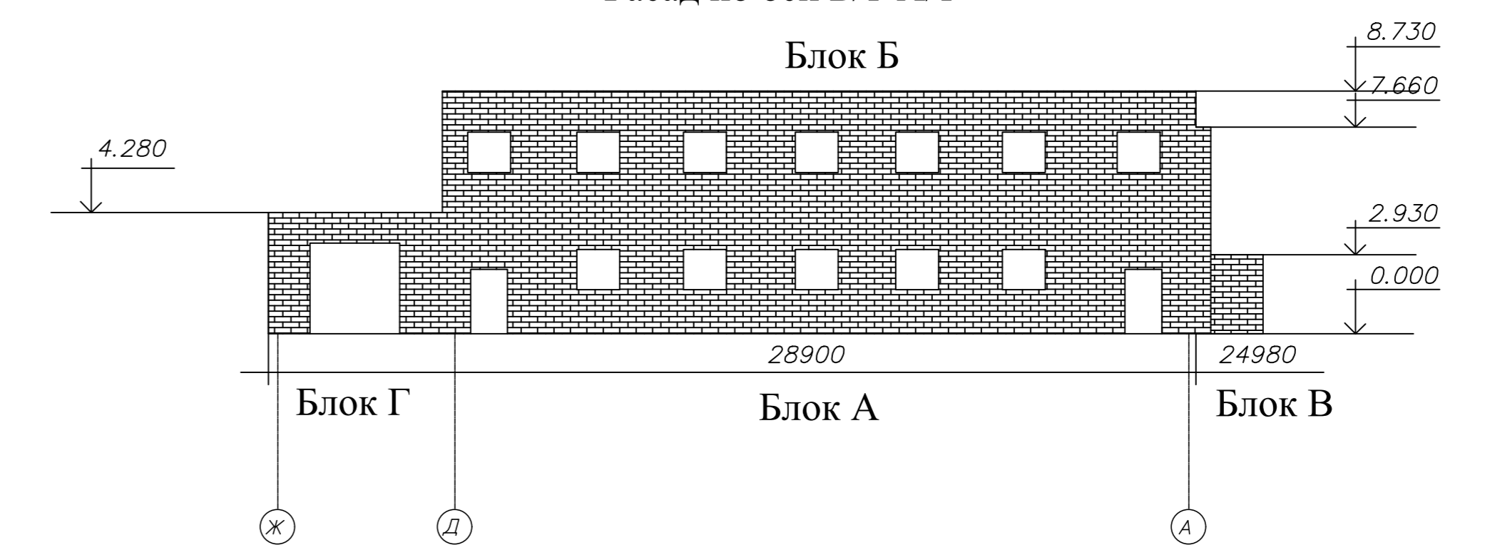
Фасад по оси Б/1-А/1
