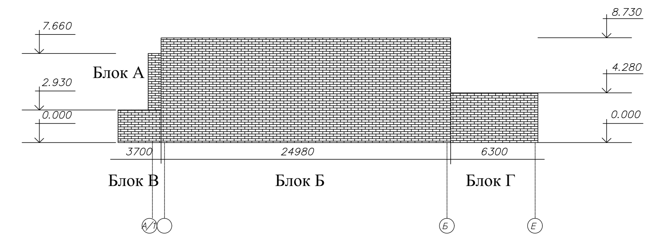
Фасад по оси А/1-Б/1
