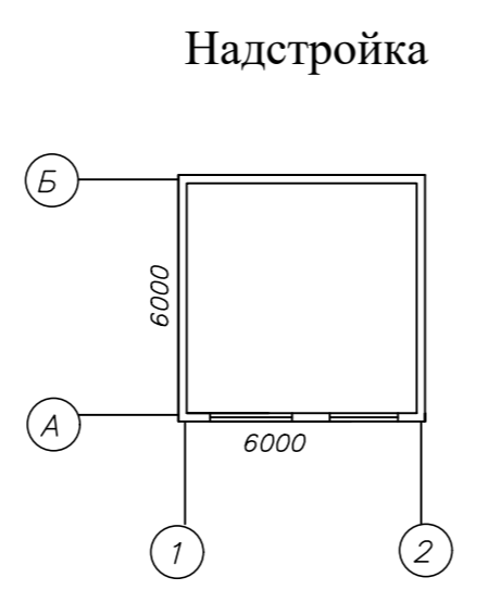
План на отм. 17.0
