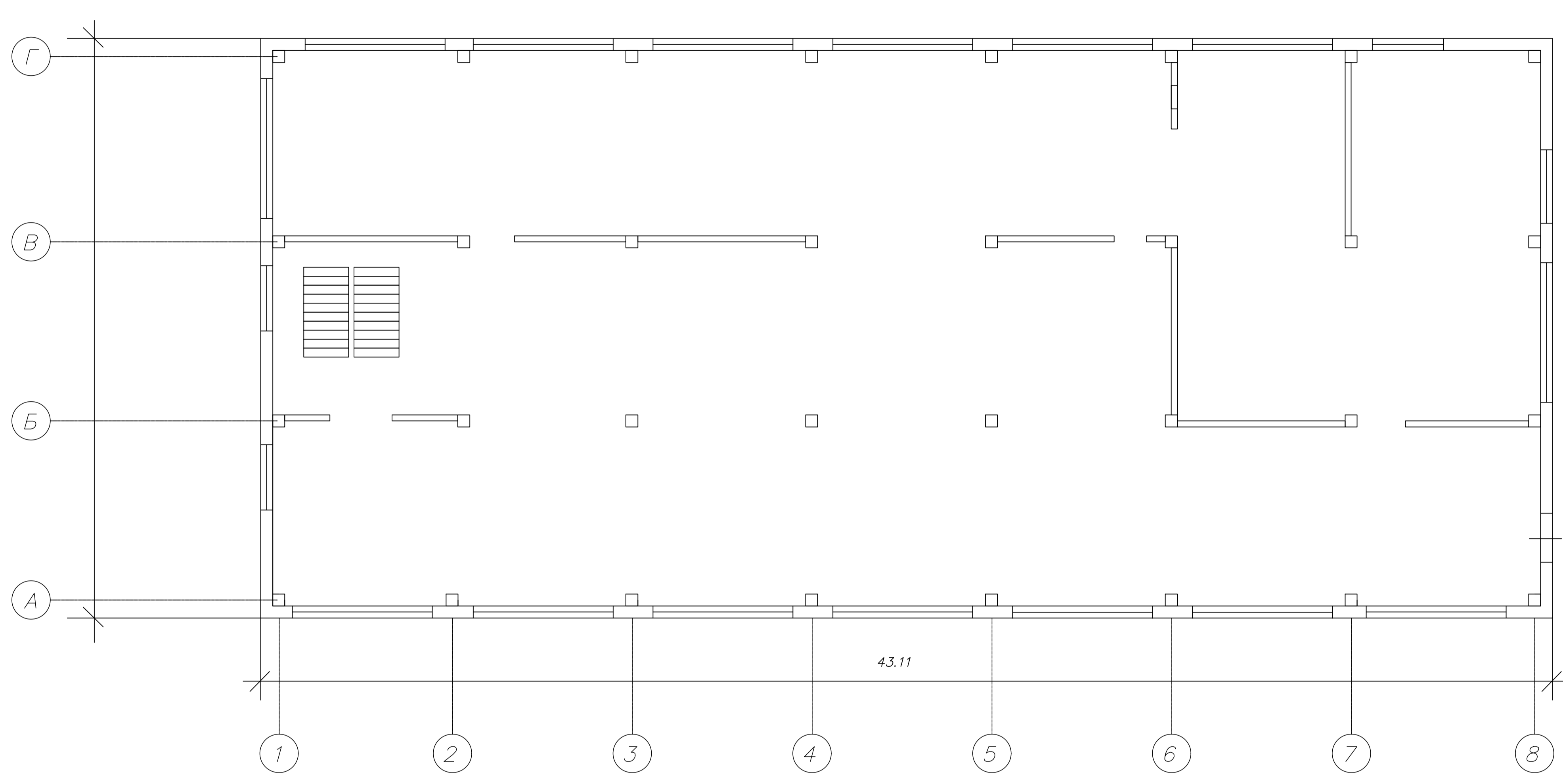
План на отм. 3.000
