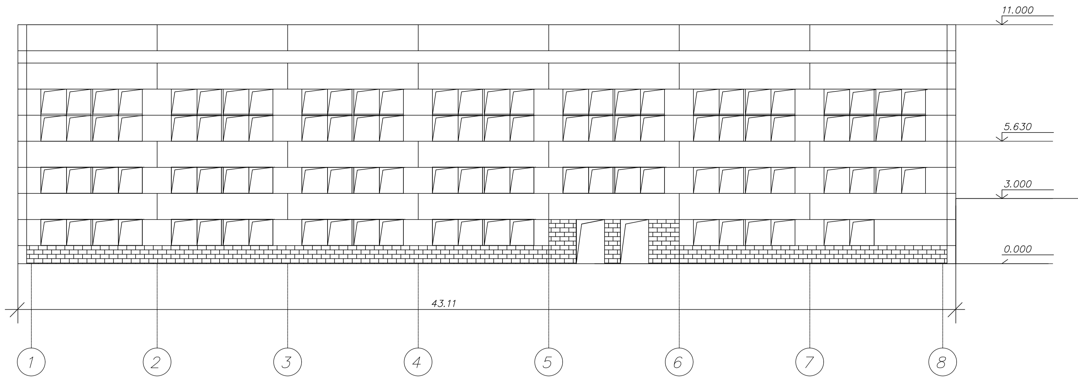
Фасад по оси 1-8
