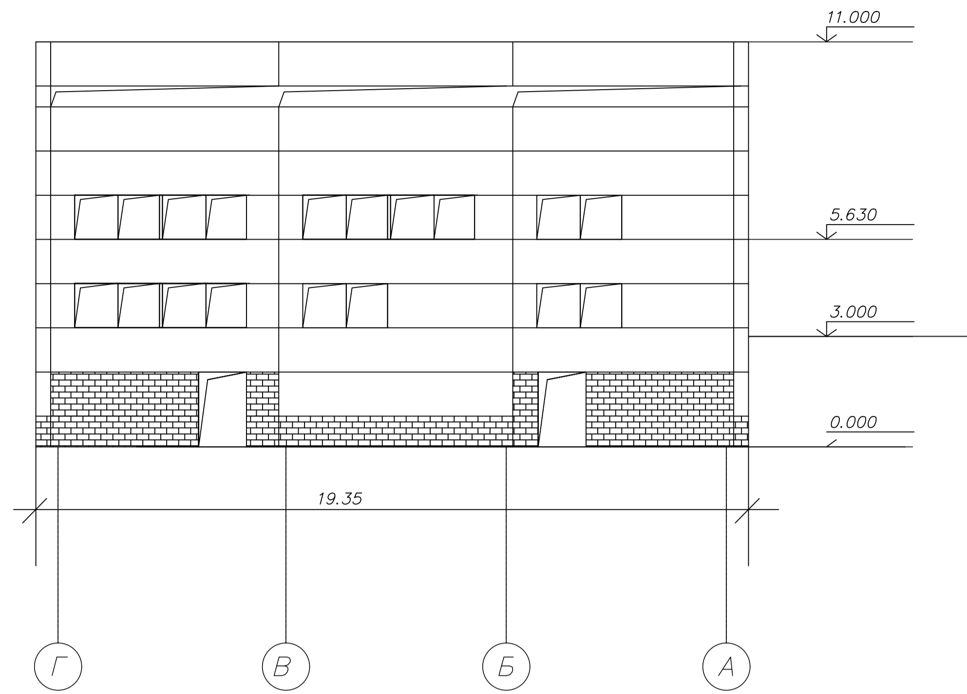
Фасад по оси Г-А
