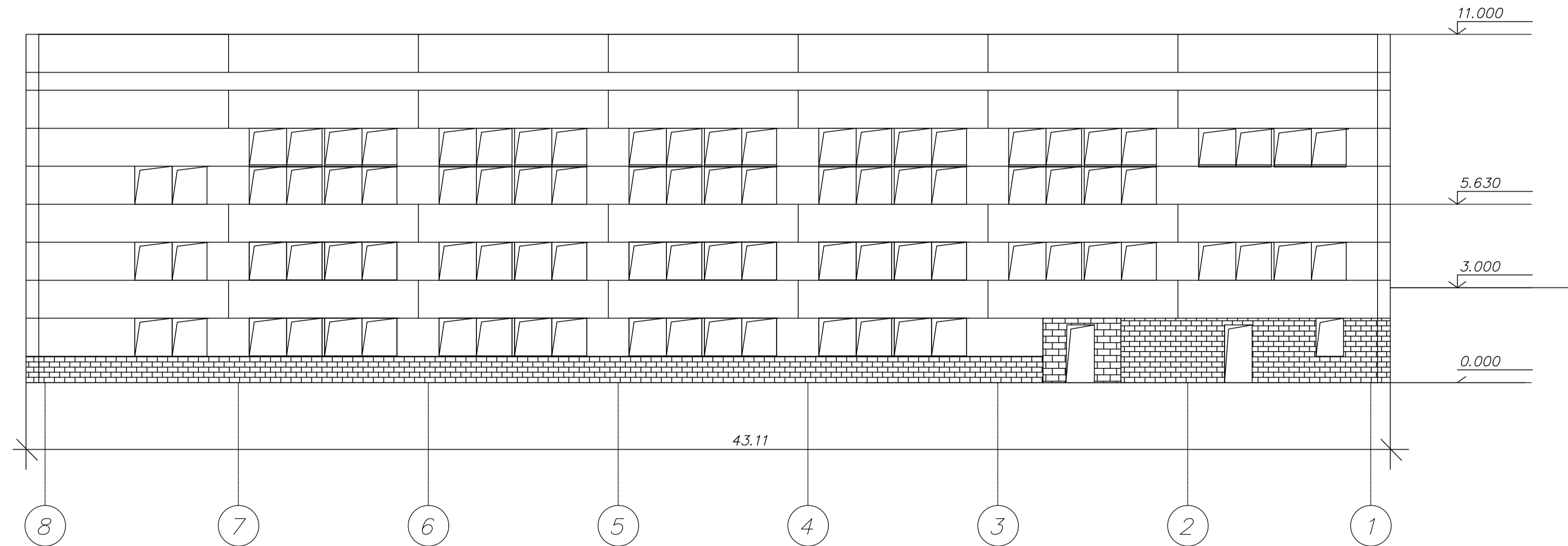
Фасад по оси 8-1
