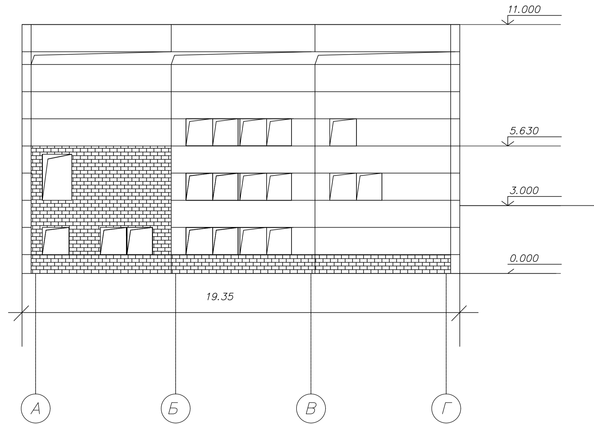
Фасад по оси А-Г
