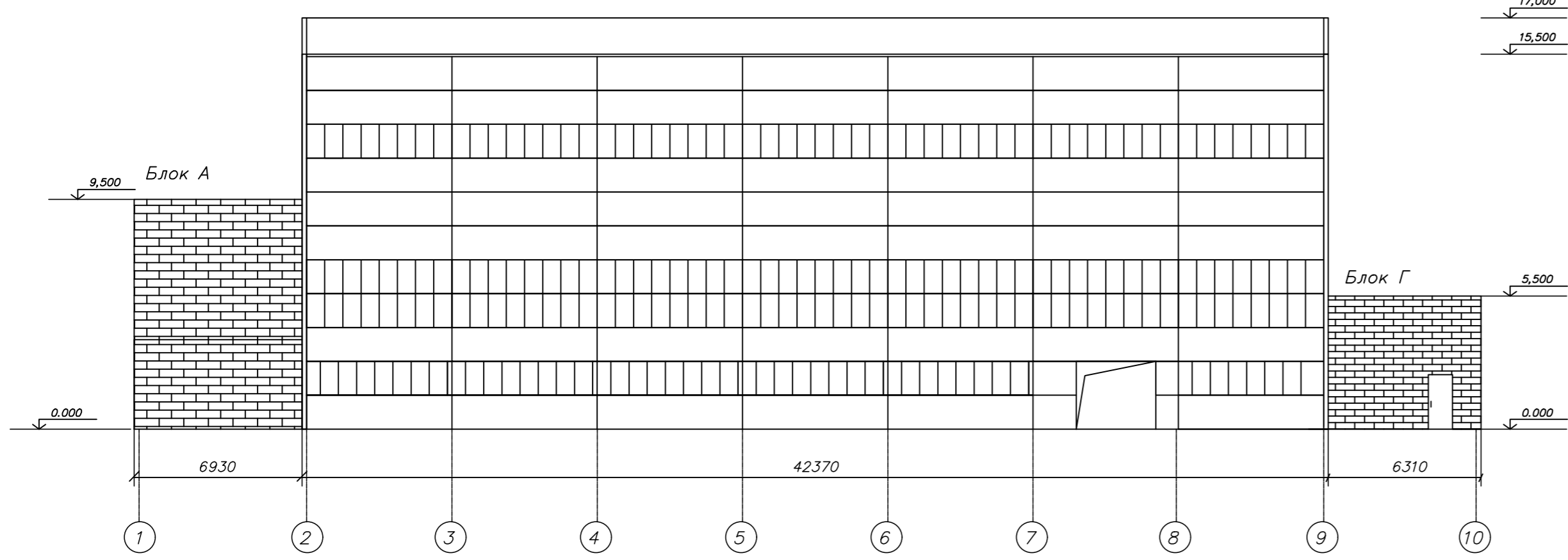
Фасад по оси 1-10 Блок Б
