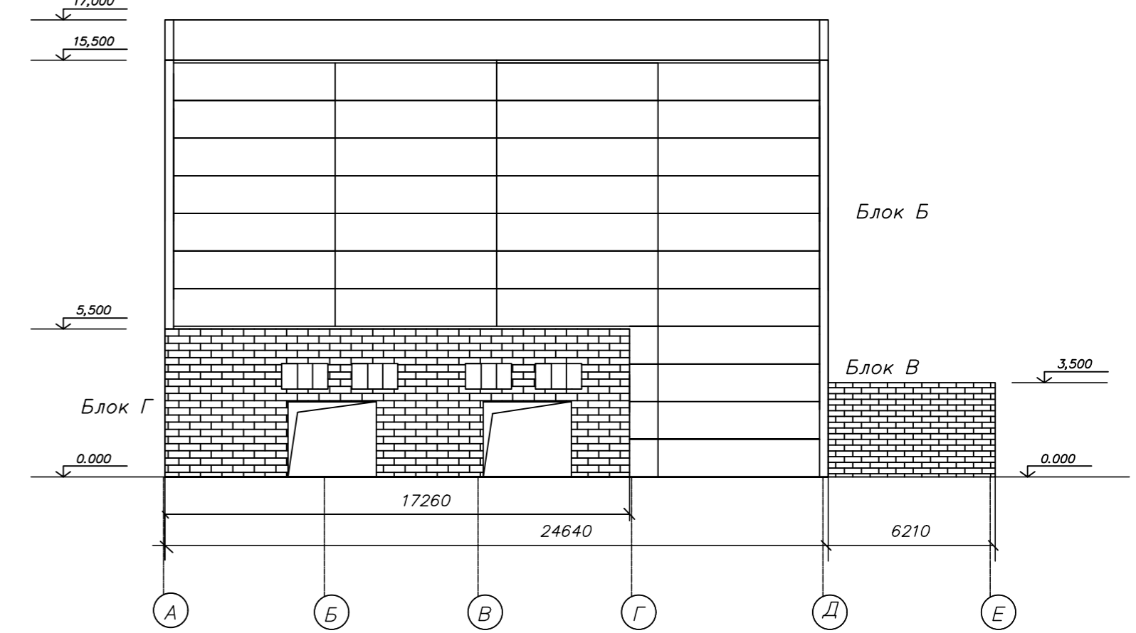
Фасад по оси А-Е
