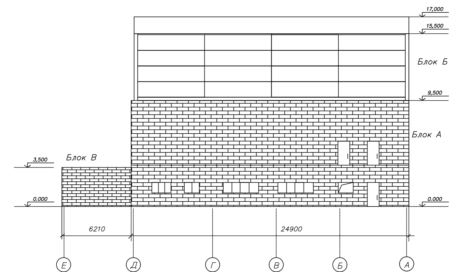
Фасад по оси Е-А
