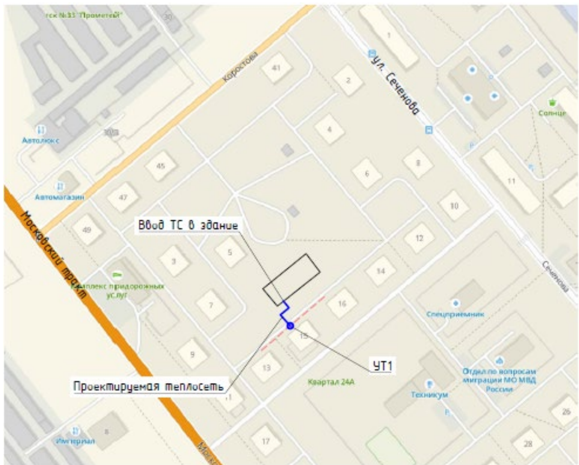
Рис. 4.1. Ситуационный план тепловой сети
