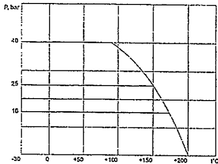
Диаграмма давление-температура
