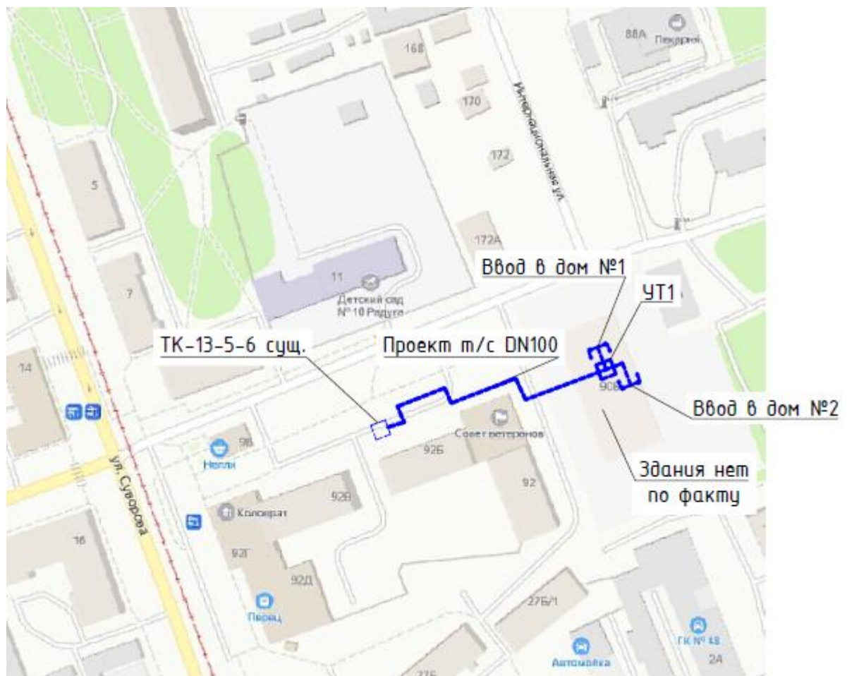
Рис. 4.1. Ситуационный план тепловой сети
