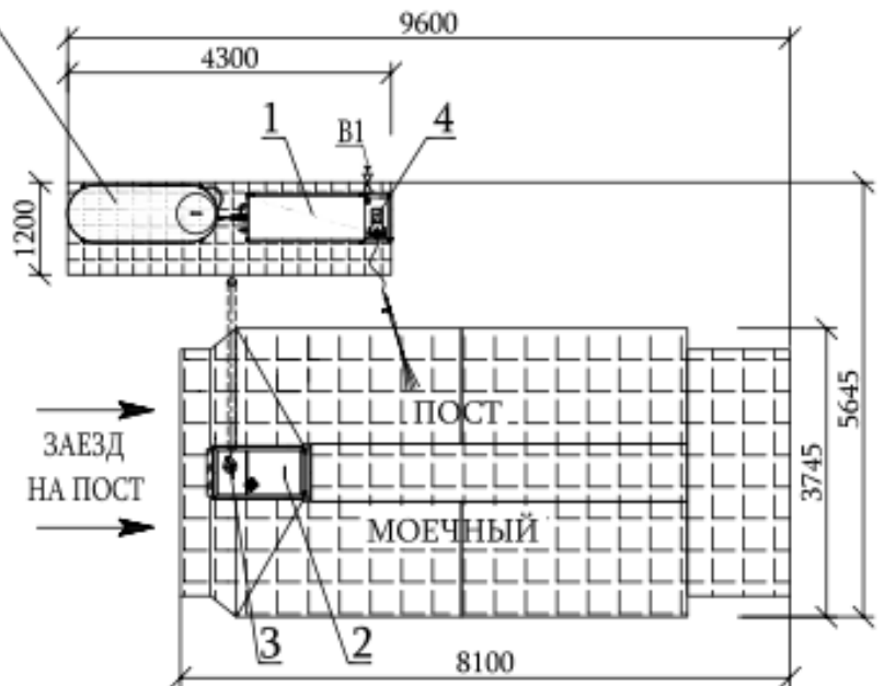
Рис.1. Схема устройства и расположения технологического оборудования.
